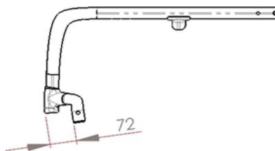
Ángulo standard y posición de la rueda adelantada, ideal para una mayor estabilidad frontal
