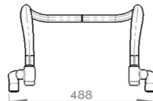
Ángulo más cerrado y posición de la rueda retrasada, lo que reduce la anchura delantera de la silla y facilita la maniobrabilidad en espacios confinados
