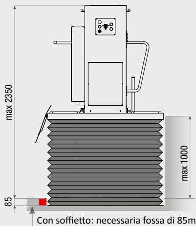
VISTA FRONTALE: ingombro pedana al piano alto con soffietto
