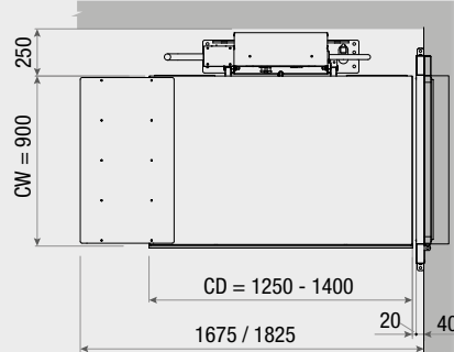
VISTA DALL'ALTO: ingombro max con pedana aperta
